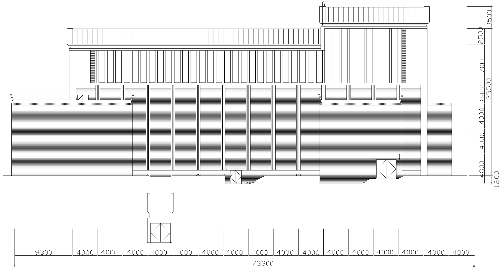
東側立面図
