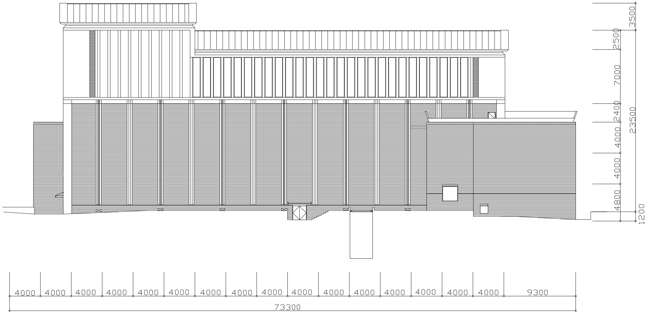
西側立面図
